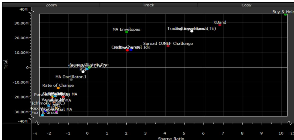
Ilustración 76: Estrategias sin optimizar Allstate
