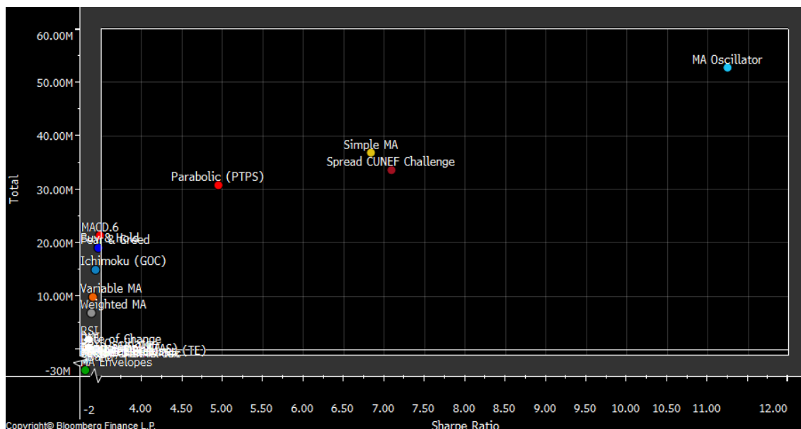
Ilustración 72: Estrategias sin optimizar Lukoil
