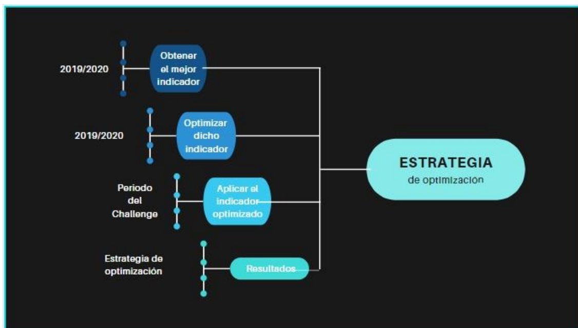
Ilustración 65. Gráfico explicativo de la estrategia de optimización
