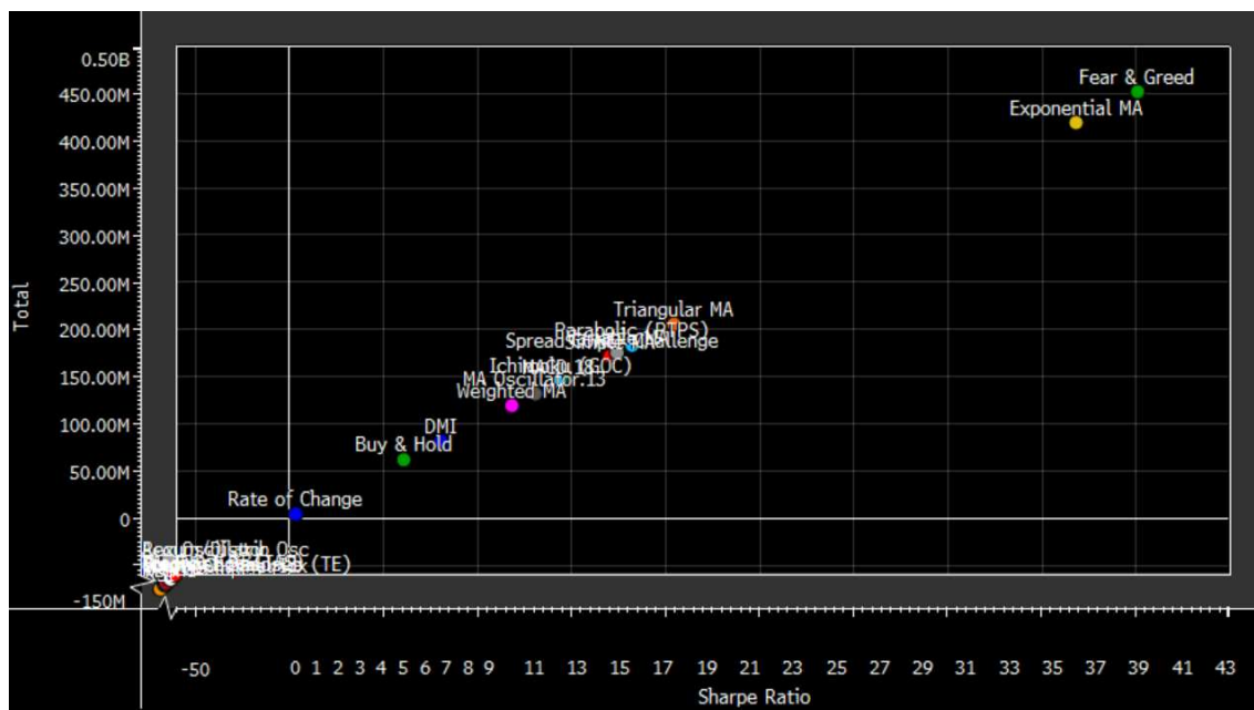
Ilustración 82: Estrategias sin optimizar Greattown Holdings
