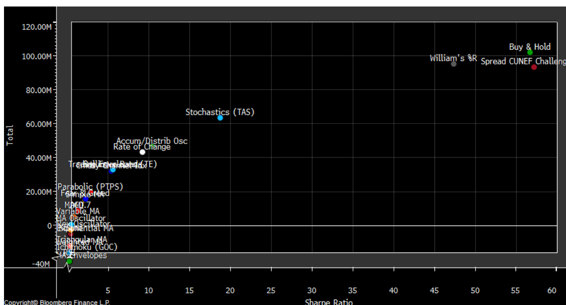
Ilustración 74: Estrategias sin optimizar COSAN
