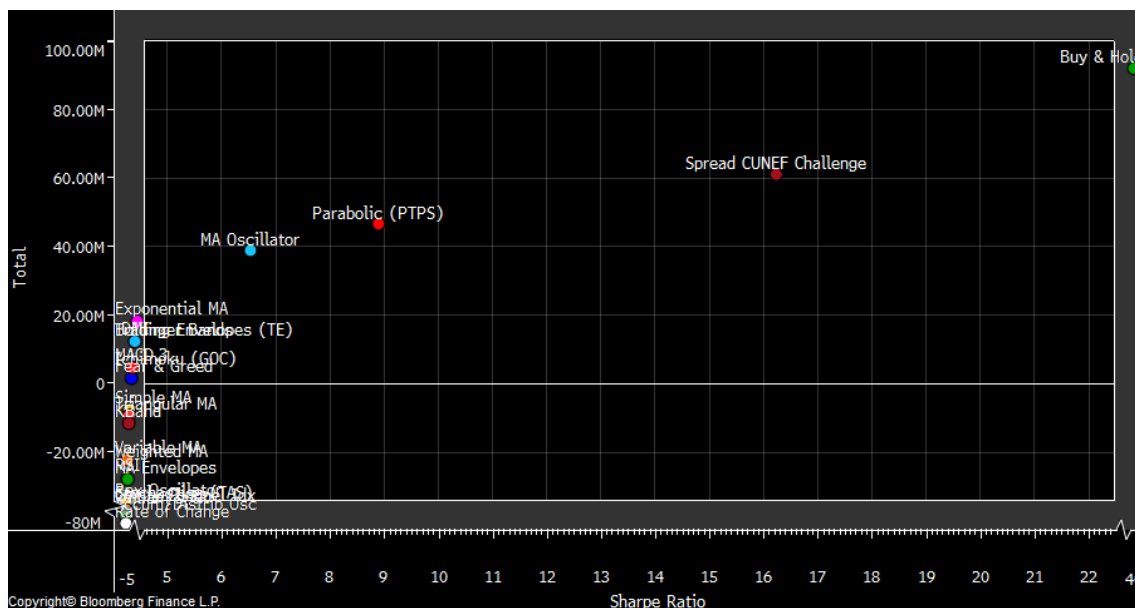
Ilustración 68: Estrategias sin optimizar FOX
