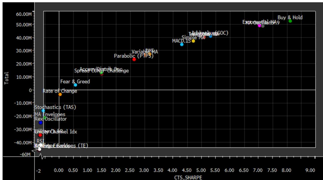
Ilustración 84: Estrategias sin optimizar Inter Rao
